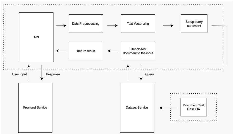
Gambar 3. 1 Desain Sistem Alur Kerja Platform
